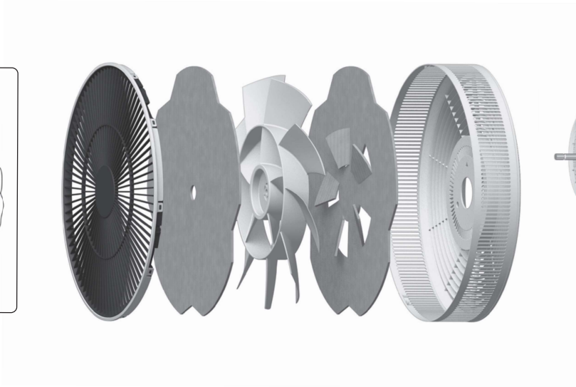
프런트 팬 가드 (1) 팬 (1) 사이드 가드 (1)
